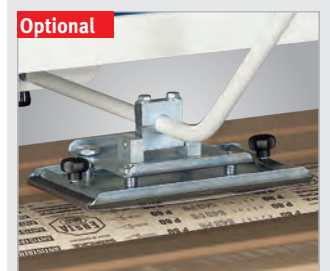
Optional Gleitschuh mit Graphitaufgabe speziell geeignet für den Feinschliff Art.-Nr. 0532PER33000 € 499,00 zzgl. USt.
