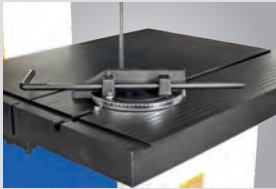
► Gehrungsanslag für Winkelschnitte ab VMBS 2013
